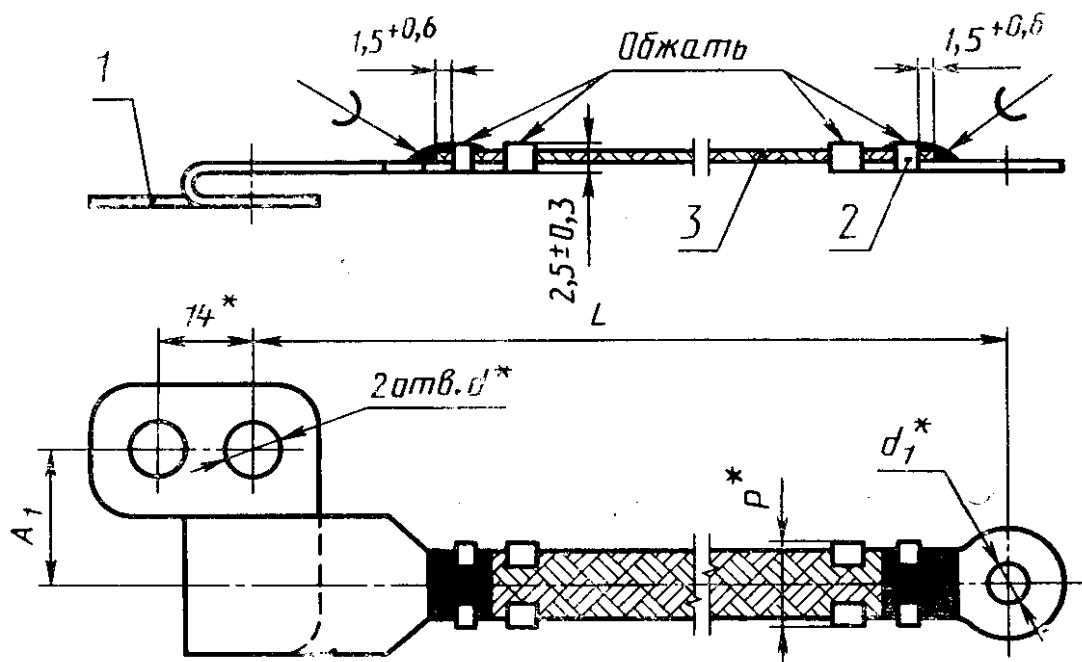
Перемычка типа К
