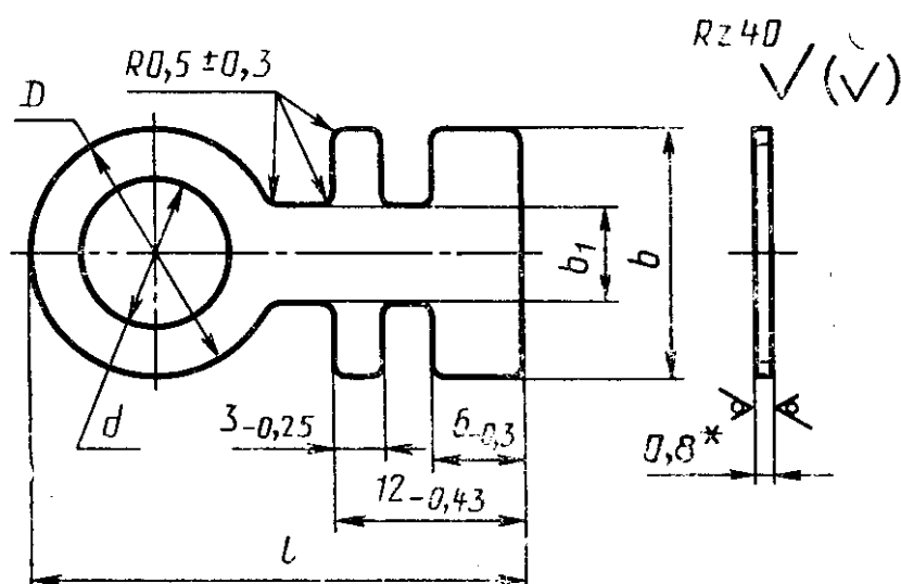
Наконечник типа А
