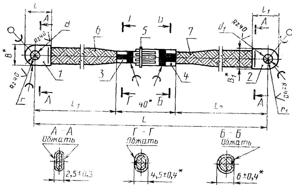
Перемычка типа И
